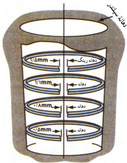
شکل ۱۲۹-۴- اندازه دهانه رینگ در محل‌های مختلف سیلندر
