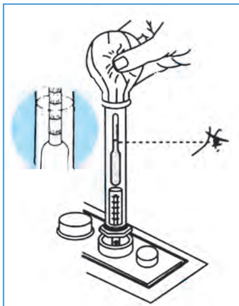
شکل ۴-۶- نحوه اندازه‌گیری غلظت محلول الکترولیت باتری با هیدرومتر دستی
