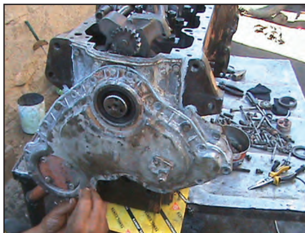
شکل ۵۹-۴- باز کردن پیچ و مهره‌های اطراف سینی جلو
