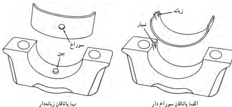
شکل ۴۳-۲- روش‌های جلوگیری از گردش یاتاقان
