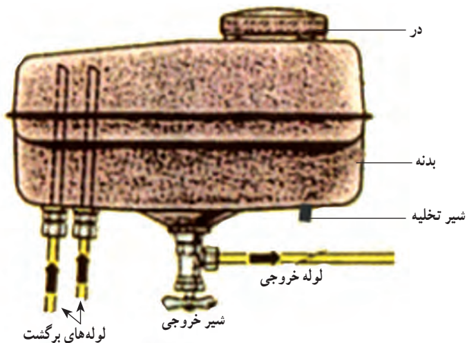
شکل ۲-۴- اجزای باک
