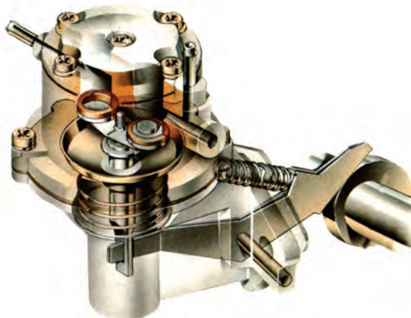
شکل ۷-۴ پمپ مقدماتی دیفراگمی
