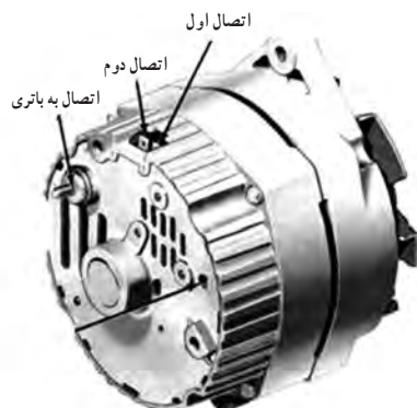
شکل ۲۶-۶- آلترناتور
