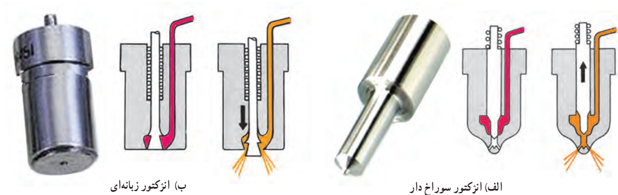
شکل ۱۷-۴- انواع انژکتور
