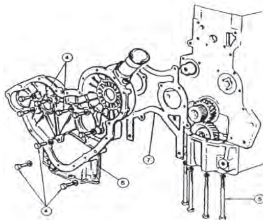
شکل ۷۵-۴- محفظه جلو موتور باز شده
