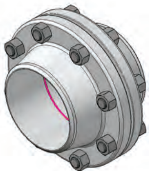
شکل ۳-۱- کاربرد پیچ و مهره برای اتصال
