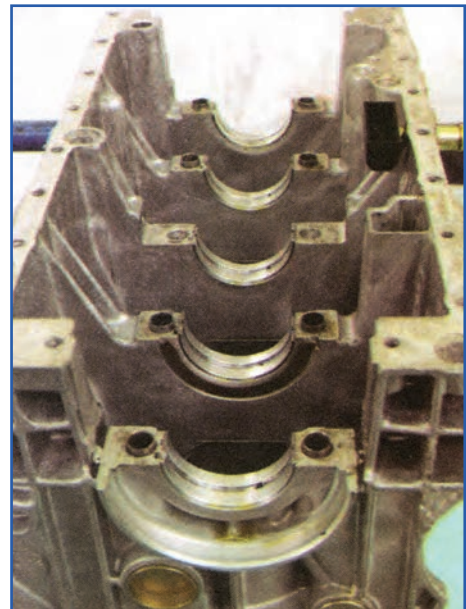
شکل ۱۸۶-۴ یاتاقان‌های ثابت در محل خود روی بدنه سیلندر
