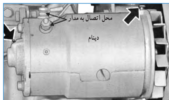
شکل ۲۵-۶- دینام
