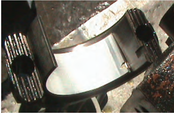
شکل ۸۶-۴- جا زدن زبانه یاتاقان در شیار کپه یاتاقان
