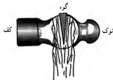
شکل ۷۵-۳- اتصال چکش به دسته
