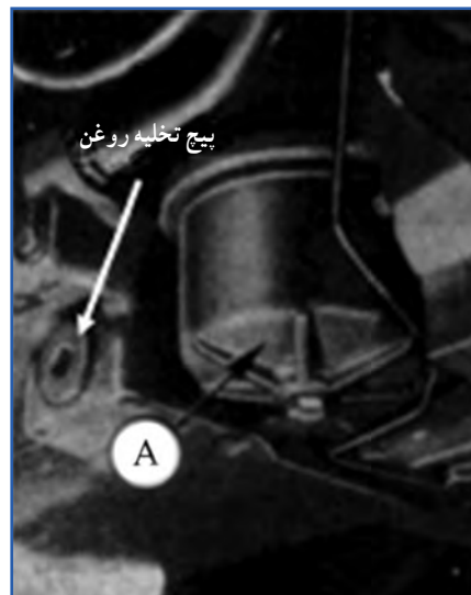
شکل ۵۷-۷ صافی روغن هیدرولیک در تراکتور جان‌دیر
