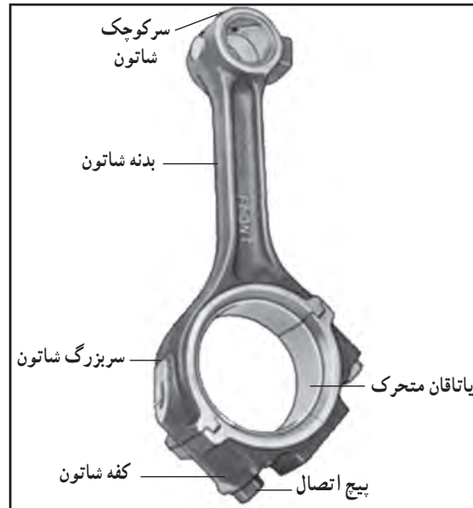
شکل ۲۸-۲- اجزای شاتون
