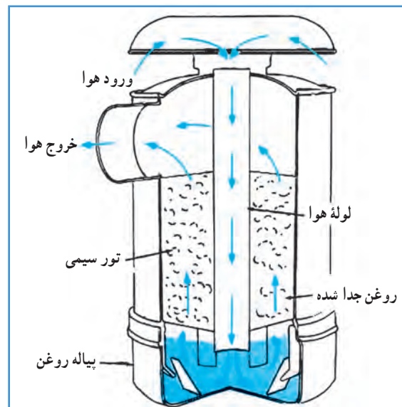
شکل ۹-۵- مسیر عبور هوا در صافی روغنی
