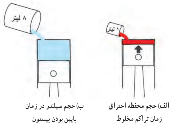
شکل ۳-۱- نسبت تراکم ۱:۸
