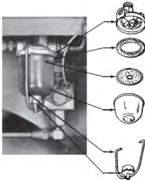
شکل ۱-۴- پیاله رسوب گیر
