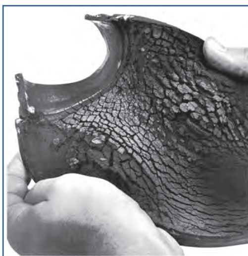
شکل ۳۹-۳- پوسیدگی شیلنگ از داخل
