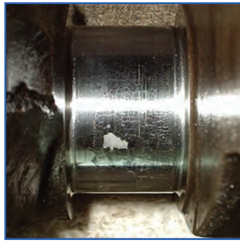
ب) پوسته کردن لایه سخت لنگ
