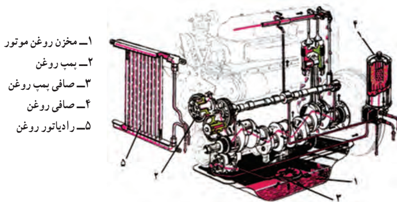
شکل ۹-۷- مدار روغن کاری موتور تراکتور U650M با مدار رادیاتور روغن
