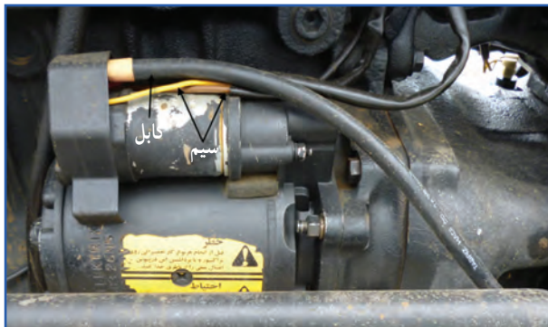
ب) سیم و کابل متصل به استارت تر شکل ۳-۷ – سیم‌های متصل به استارت تر و جلو داشبورد
