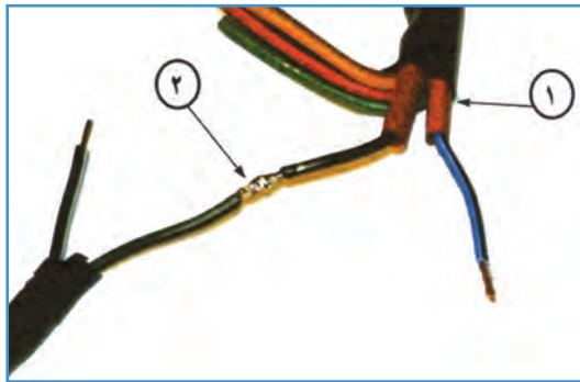
شکل ۶۶-۶- نحوه لحیم کاری سیم‌ها
