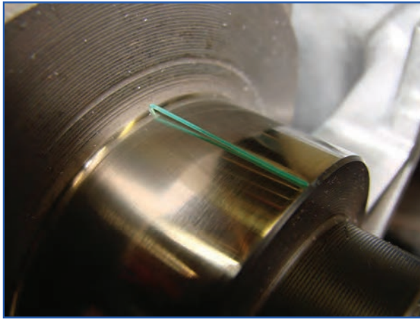
شکل ۱۷۵-۴- قرار دادن پلاستیکی گیج روی محور
